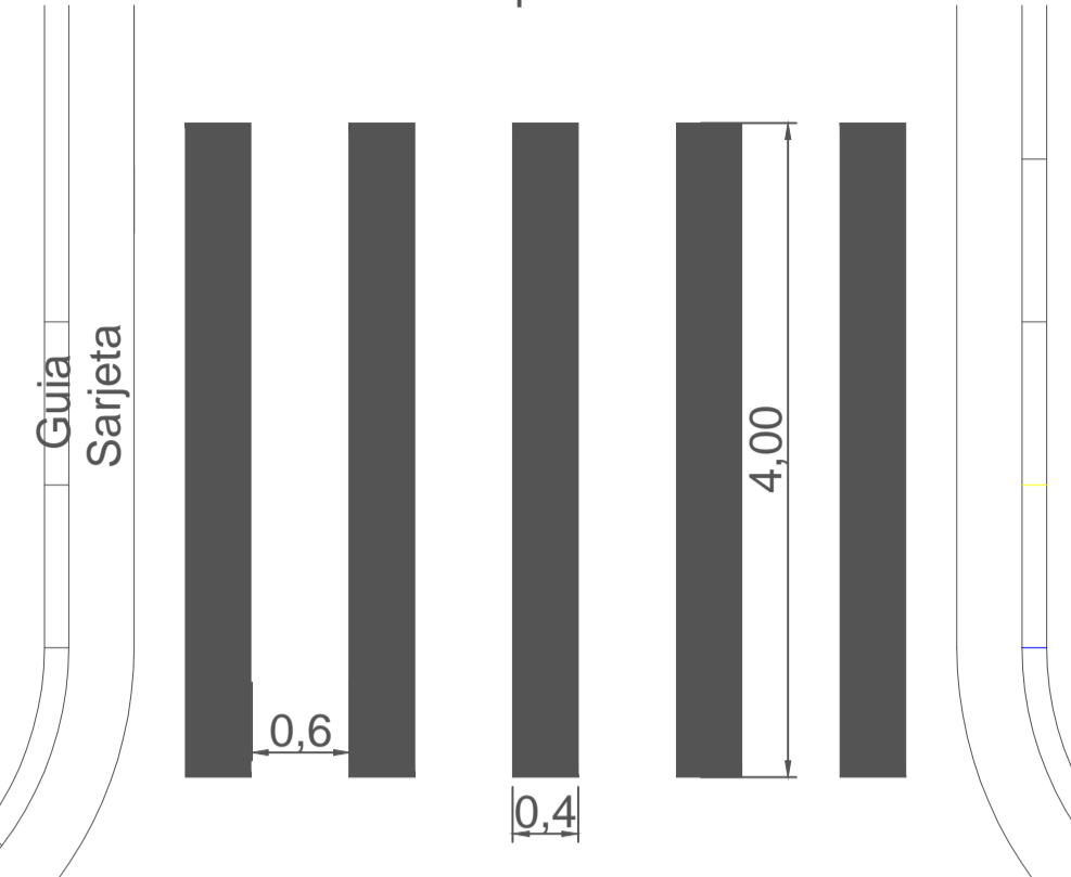
Detalhe 3 Faixa de pedestre cor branca
