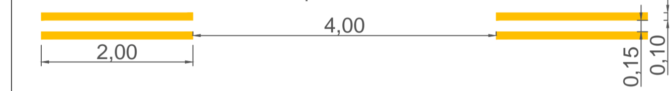
Detalhe 3 Faixa de pedestre cor branca
