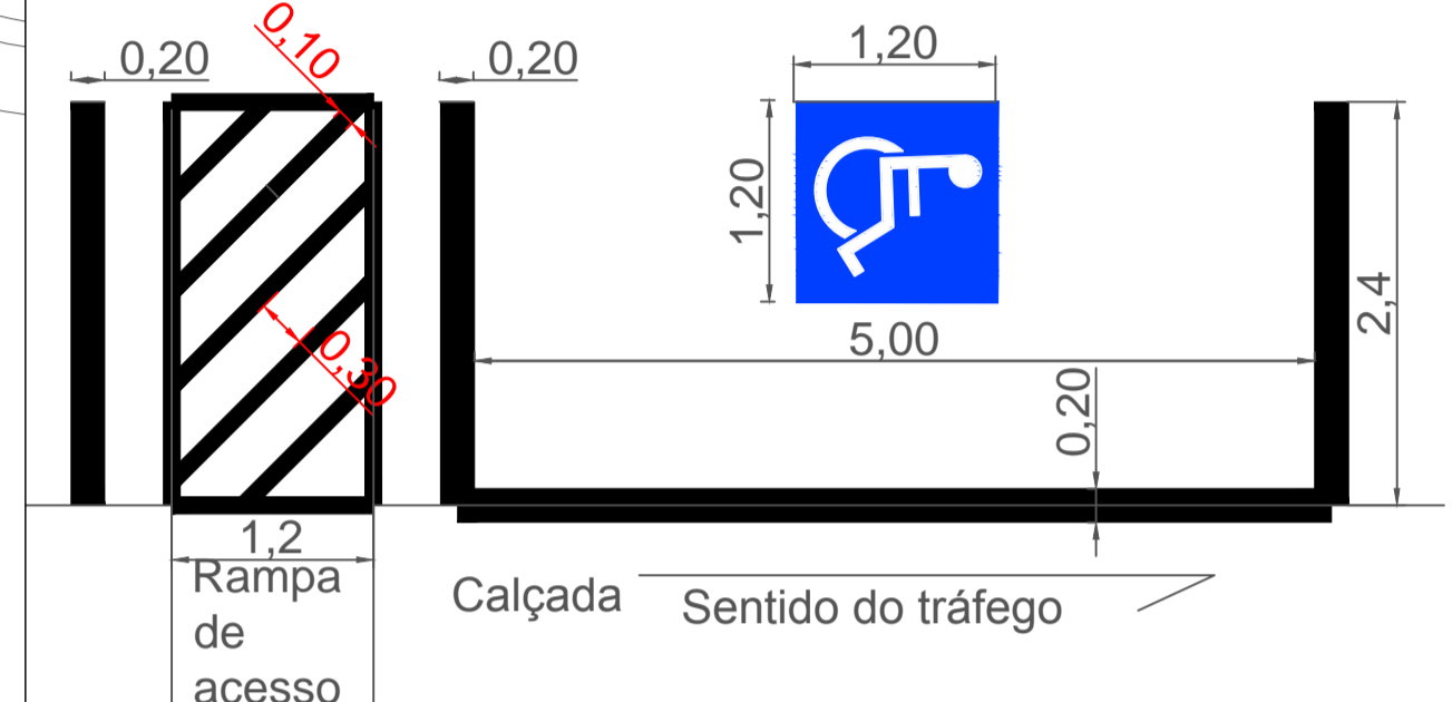
Detalhe 7 Linha de retenção cor branca
