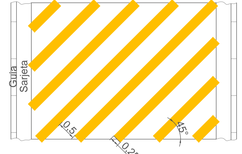
Detalhe 4 Pintura de lombada cor amarela
