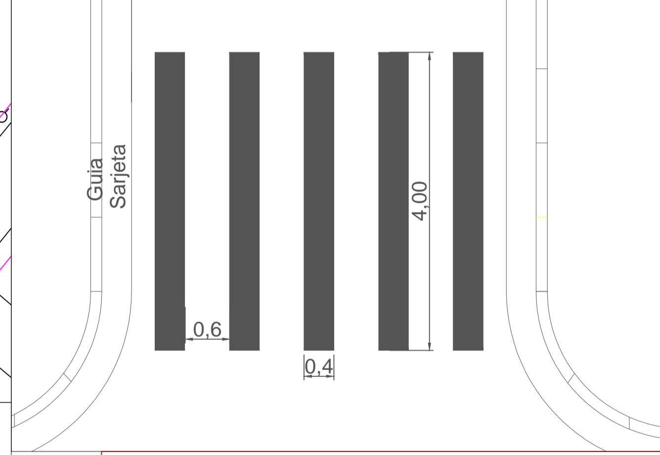
Detalhe 3 Faixa de pedestre cor branca
